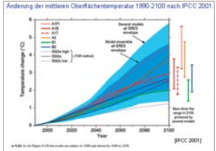
Quelle: Änderung der mittleren Oberflächentemperatur 1990-2100 nach IPCC 2001
